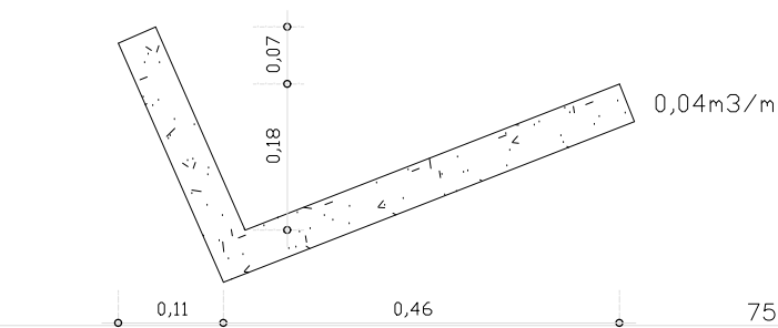
DET. CANALETA TRIANGULAR EXIST. ESC: 1:10 MEDIDA EM METROS
