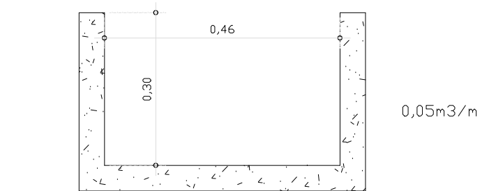
DET. CANALETA RETANGULAR EXIST. ESC: 1:10 MEDIDA EM METROS
