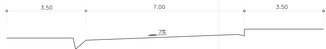
PERFIL TRANSVERSAL DA RUA DAS MANGUEIRAS (EXISTENTE)
