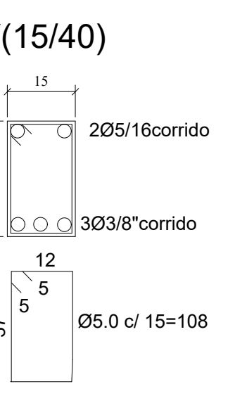
VIGAS
