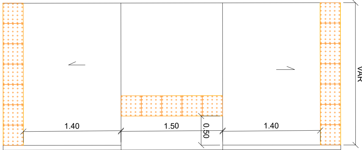
PLANTA BAIXA
