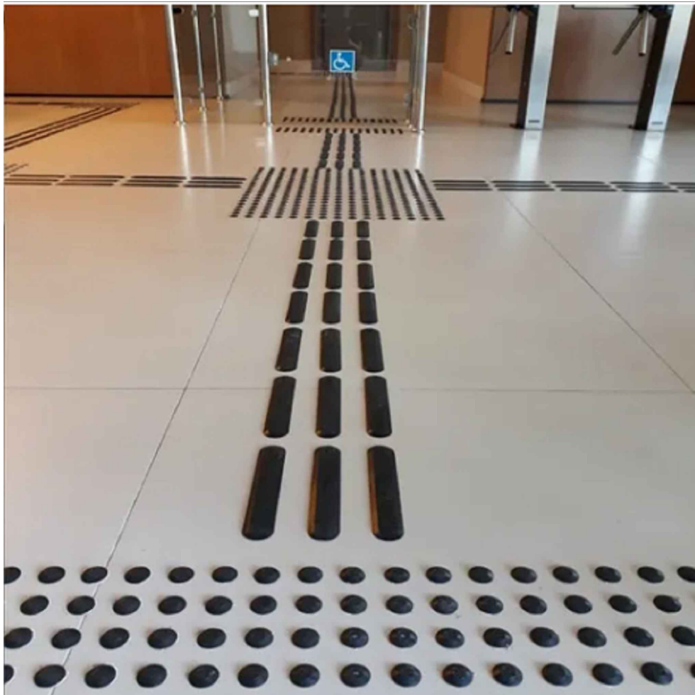
MODELO1 – PISO PODOTÁTIL INTERNO
