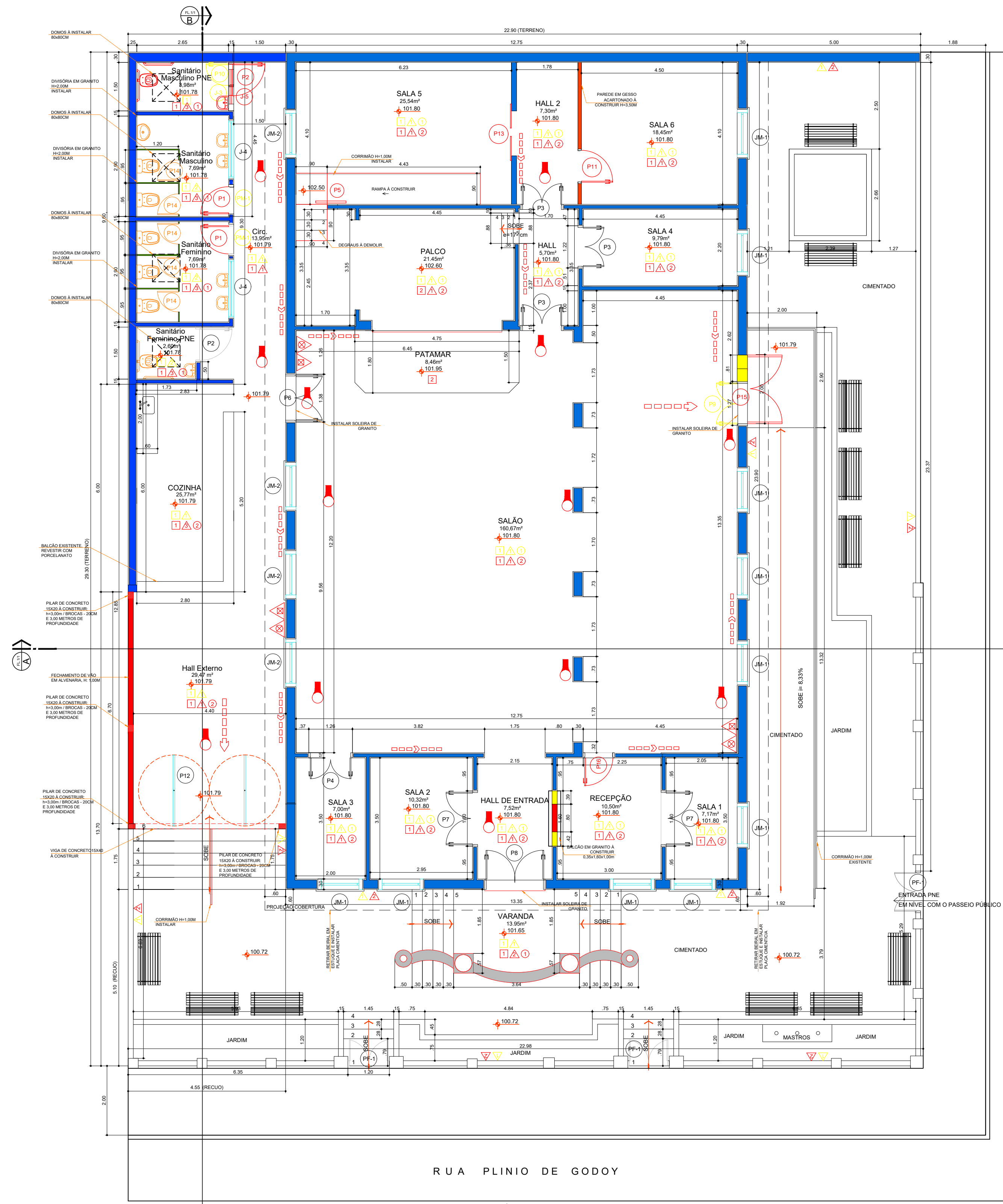
PLANTA BAIXA
