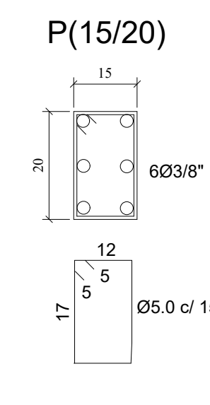
PILARES
