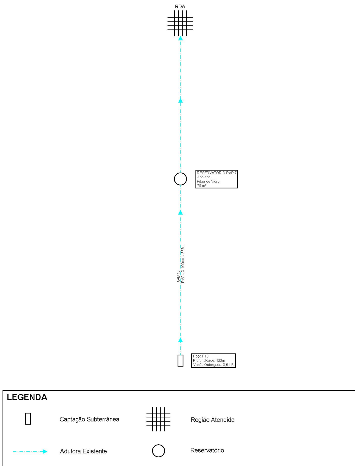
Figura 4.5 – Croqui do Sistema de Abastecimento de Água Existente –Bairro Vale Florido.
