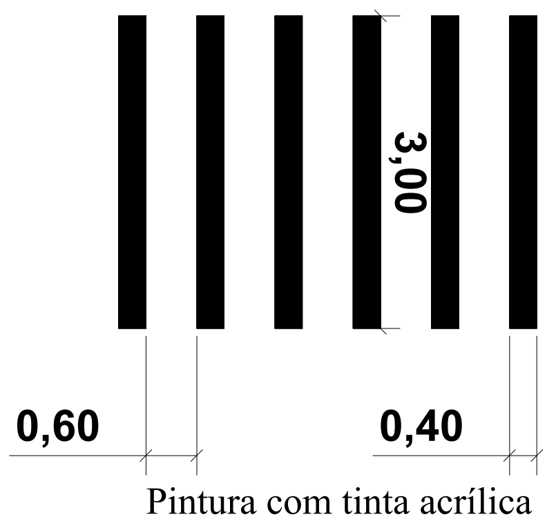
Pintura com tinta acrílica
